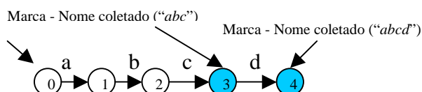
Figura 4 – Configuração do autômato p/string “abcd”
