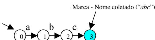
Figura 3 – Configuração do autômato p/ string “abc”
