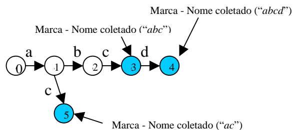
Figura 5 – Configuração do autômato adaptativo adicionando o string “ac”
